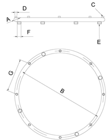
Dimensions/ Dimensiones
